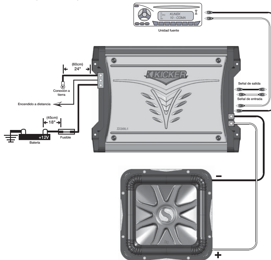
Funcionamiento por un canal (monofónico) Impedancia mínima de 2 Ω en puente
